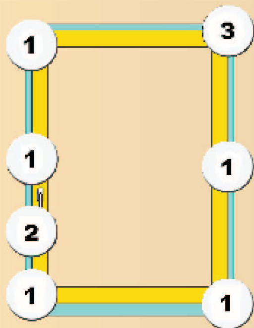
Punti di lubrificazione della ferramenta sulla finestra
